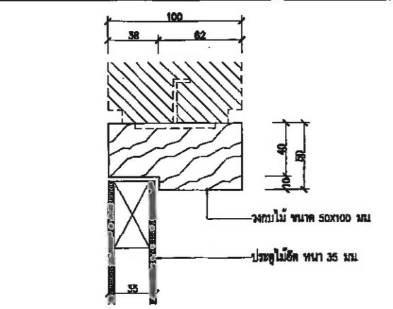
แบบขยายรูปตัด 4
