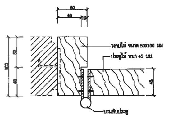
แบบขยายรูปตัด 7
