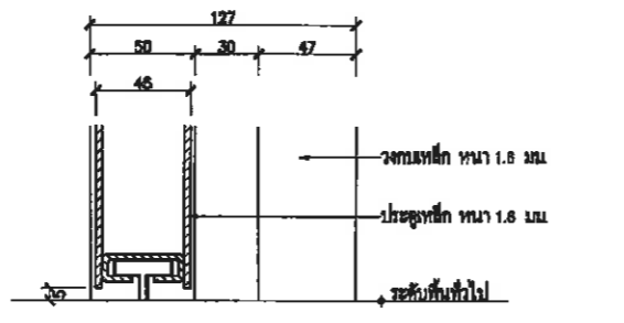
แบบขยายรูปตัด ⑤
