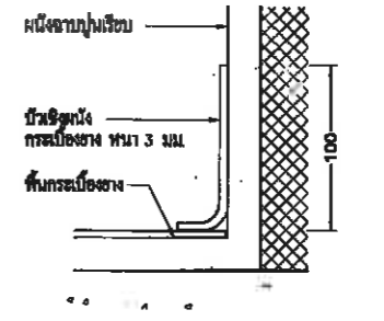
แบบขยายบัวพื้น B8 มาตราส่วน 1: 2.5 AT A1 1: 5 AT A3
