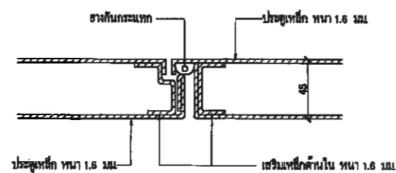
แบบขยายรูปตัด ③
