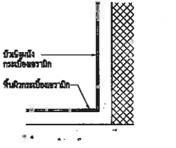
แบบขยายบัวพื้น B7 มาตราส่วน 1: 2.5 AT A1 1: 5 AT A3
