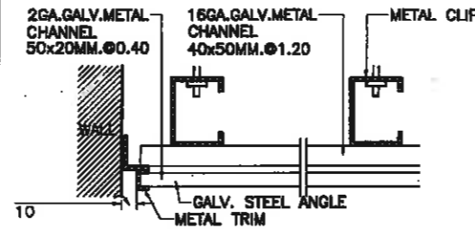
GYP. BOARD CEILING 7 มาตราส่วน 1 : 2.5 AT A1 1 : 5 AT A3
