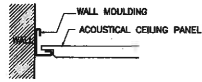
TYP. SUS.AC.CEILING 1 มาตราส่วน 1 : 2.5 AT A1 1 : 5 AT A3
