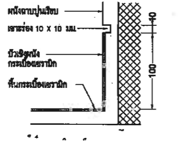
แบบขยายบัวพื้น B6 มาตราส่วน 1: 2.5 AT A1 1: 5 AT A3
