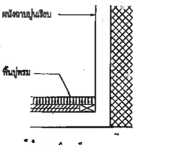
แบบขยายบัวพื้น B4 มาตราส่วน 1: 2.5 AT A1 1: 5 AT A3
