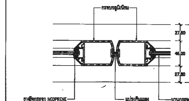
แบบขยายรูปตัด ⑧
