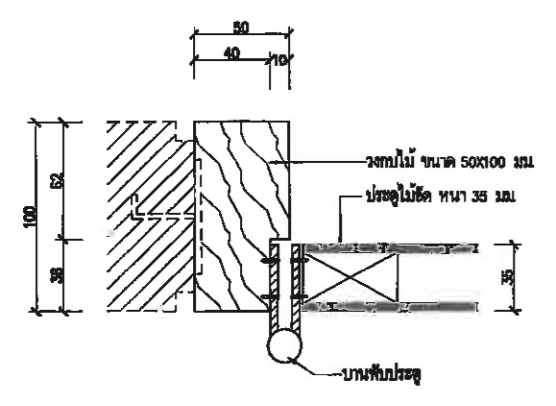
แบบขยายรูปตัด 2
