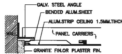
ALUM. STRIP CEILING 8 มาตราส่วน 1 : 2.5 AT A1 1 : 5 AT A3
