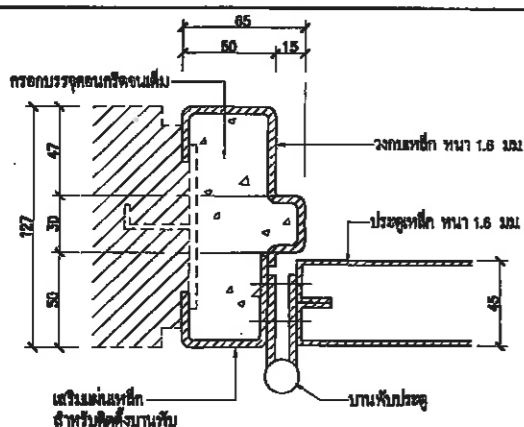
แบบขยายรูปตัด ②
