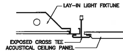
TYP. SUS.AC.CEILING 3 มาตราส่วน 1 : 2.5 AT A1 1 : 5 AT A3
