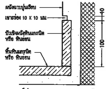
แบบขยายบัวพื้น B1 มาตราส่วน 1: 2.5 AT A1 1: 5 AT A3
