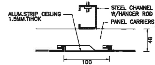
ALUM. STRIP CEILING 9 มาตราส่วน 1 : 2.5 AT A1 1 : 5 AT A3
