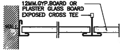
TYP. GYP. BOARD OR PLASTER GYP. BOARD EXPOSED GRID มาตราส่วน 1 : 2.5 AT A1 1 : 5 AT A3
