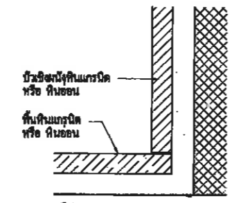
แบบขยายบัวพื้น B2 มาตราส่วน 1: 2.5 AT A1 1: 5 AT A3
