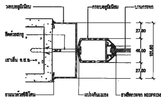
แบบขยายรูปตัด ⑦
