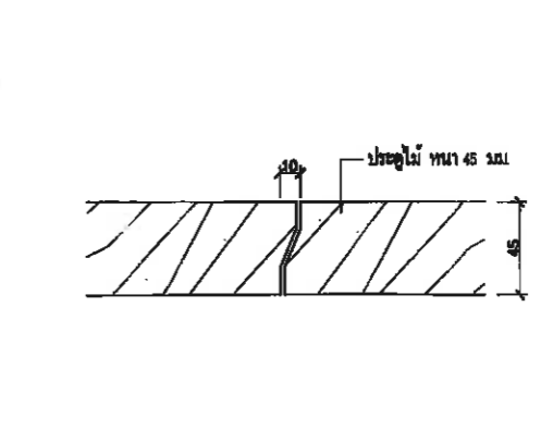
แบบขยายรูปตัด 8
