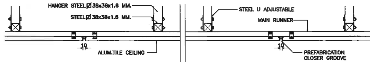
DETAIL (ALUM. TILE CEILING) 11 มาตราส่วน 1 : 5 AT A1 1 : 10 AT A3
