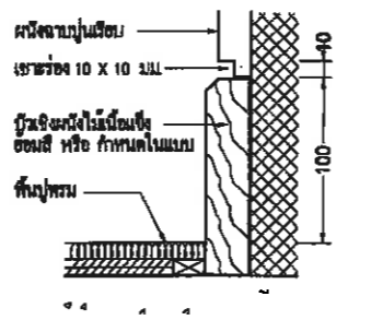
แบบขยายบัวพื้น B3 มาตราส่วน 1: 2.5 AT A1 1: 5 AT A3
