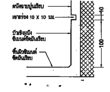
แบบขยายบัวพื้น B5 มาตราส่วน 1: 2.5 AT A1 1: 5 AT A3
