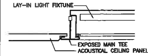
TYP. SUS.AC.CEILING 4 มาตราส่วน 1 : 2.5 AT A1 1 : 5 AT A3
