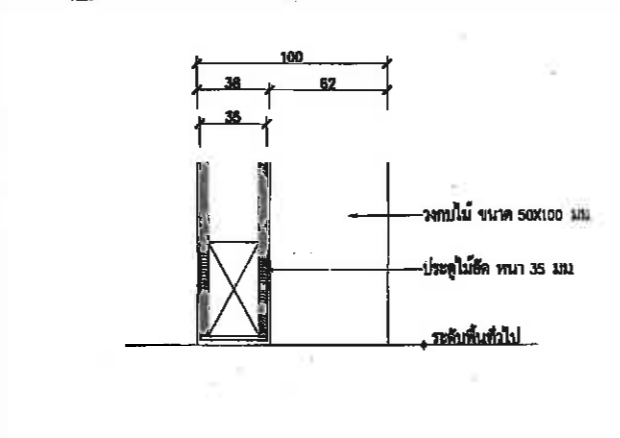
แบบขยายรูปตัด 5
